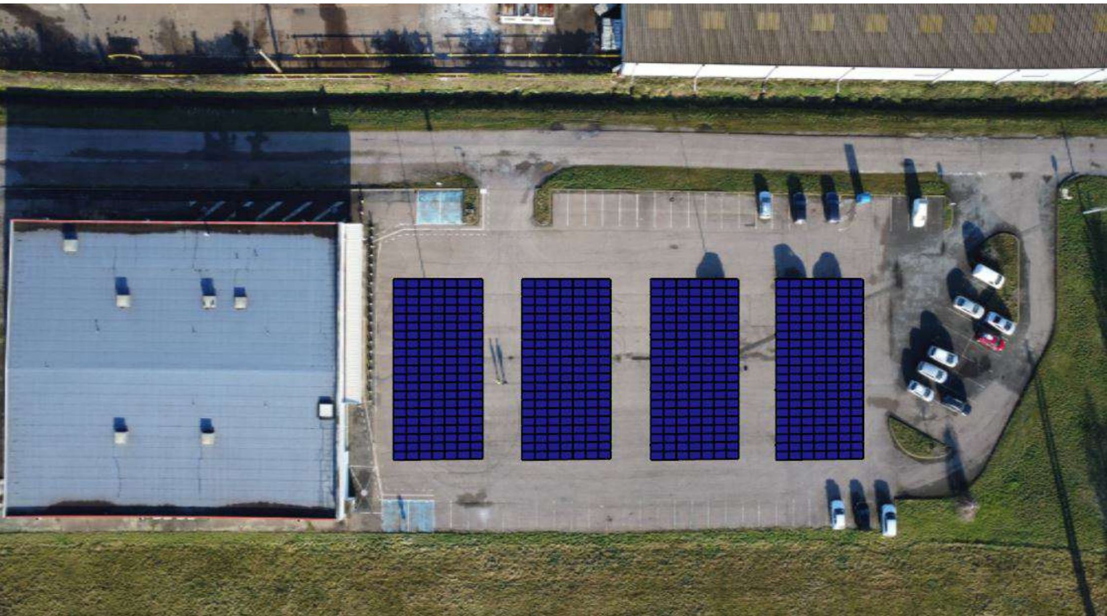
Plan implantation ombrières Pôle associatif V1
